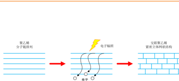
图 7：PE 电子辐照交联技术使线性分子链变为网状从而优化性能
