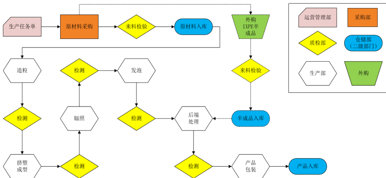
图 8：润阳科技 IXPE 材料生产环节示意图
