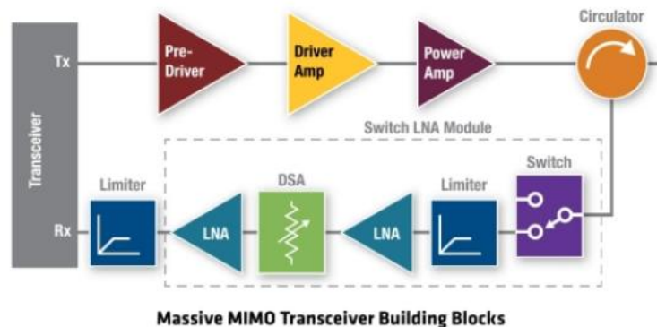
图表 27: Massive MIMO 结构示意图，环形器用于期稳定和功率放大器
