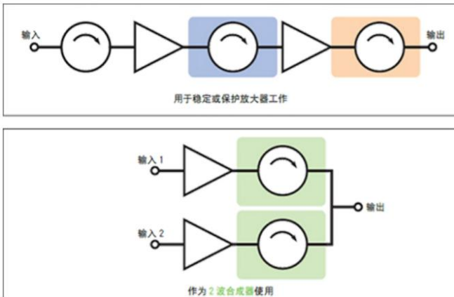
图表 28: 隔离器用于保护或稳定放大器、波合成器使用
