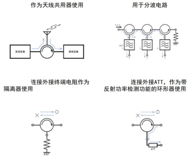
图表 29: 环形器用于天线、分波电路等功能
