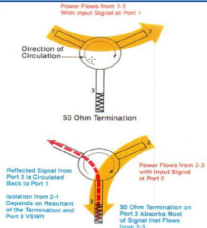
图表 26: 隔离器在端口 3 添加负载终端形成隔离器
