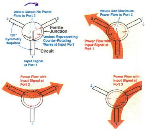
图表 25: 环形器示意图
