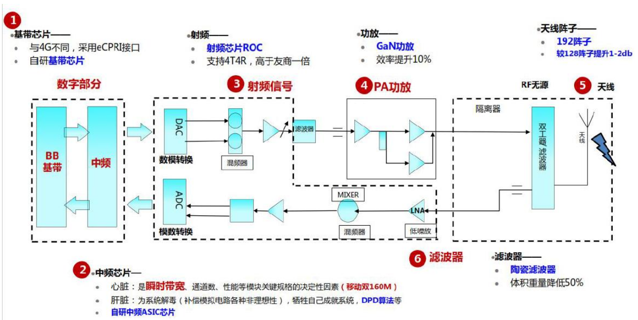
图表 20: 5G 时射频前端的变化
