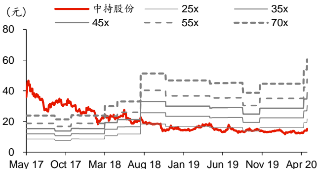
图表5: 中持股份历史 PE-Bands
