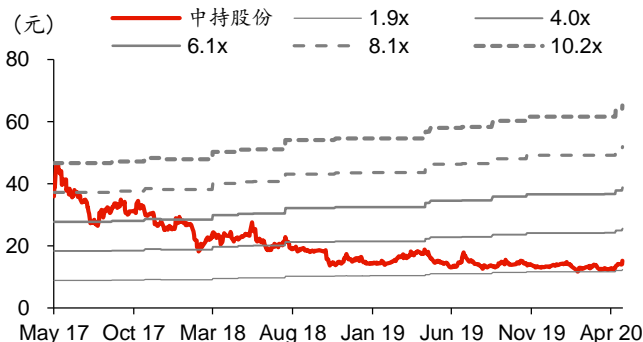
图表6: 中持股份历史 PB-Bands
