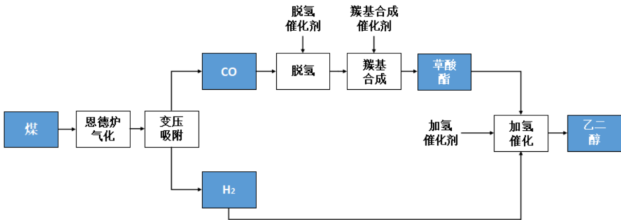
图表64：草酸酯法制乙二醇工艺流程
