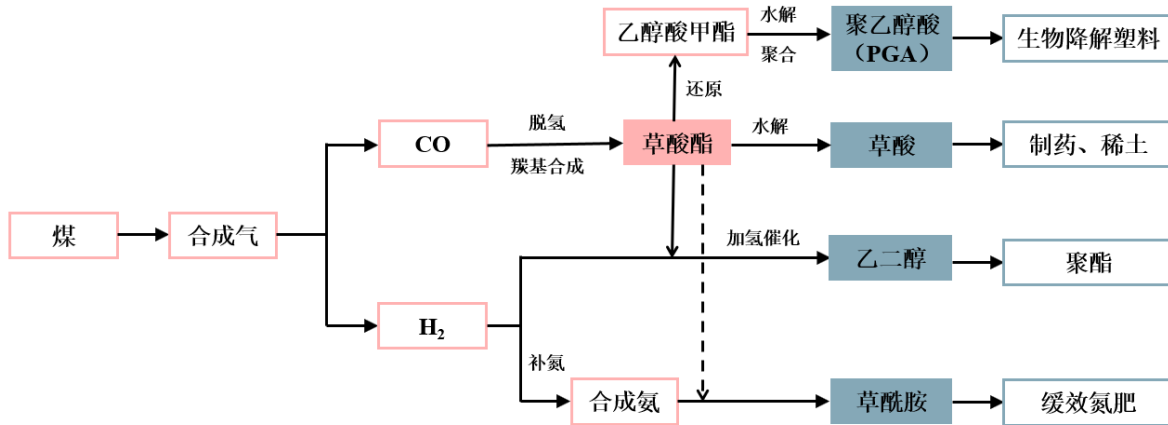
图表10：丹化科技主要产品产业链
