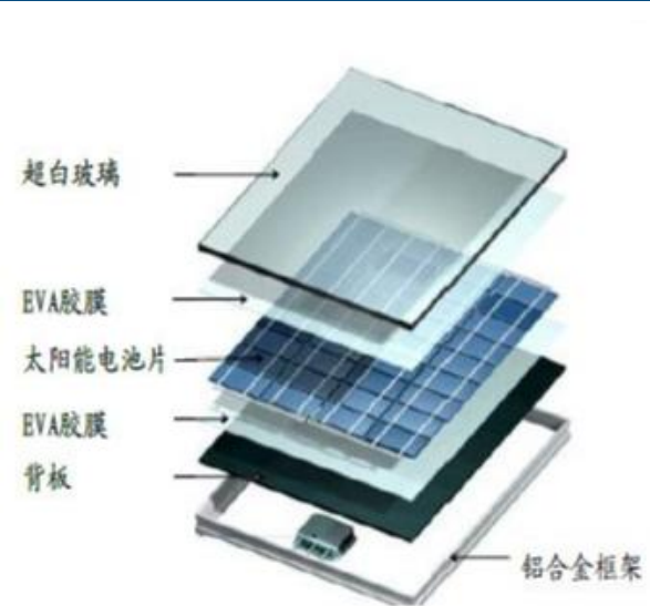
图表45: 光伏组件结构
