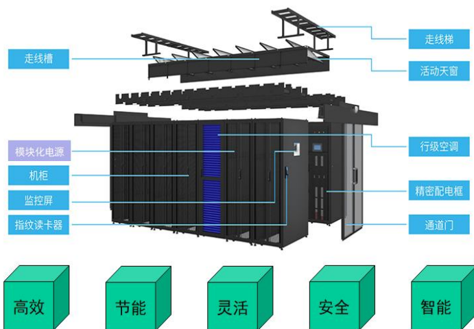
微模块数据中心示意图
