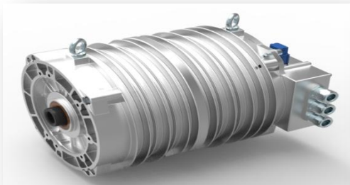
18kW交流异步电机
