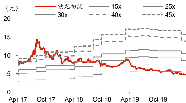
图表5: 铁龙物流历史 PE-Bands
